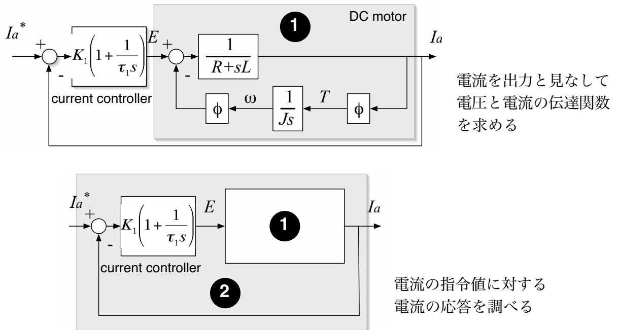
図 2: 電流制御部分の取り出し
