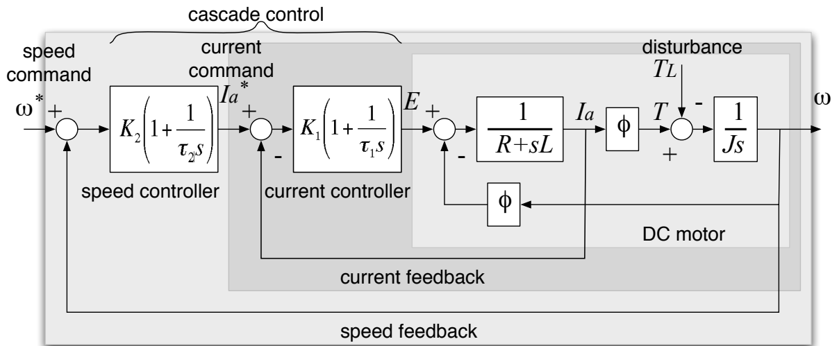
図 1: 直流機速度制御系全体図
