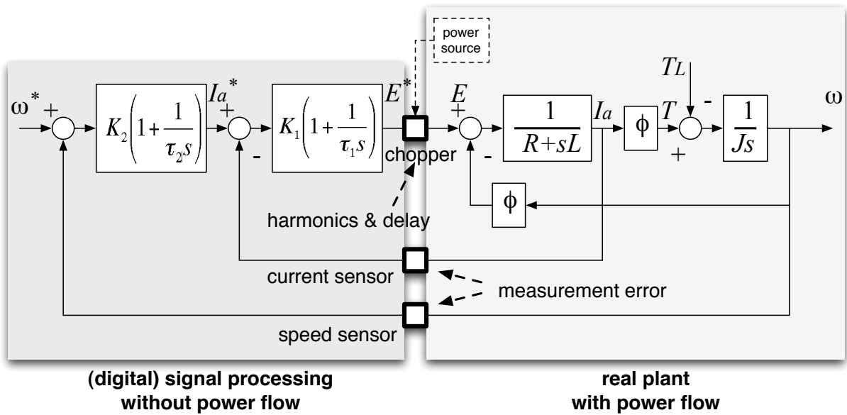
図 5: 実システムとの対応
