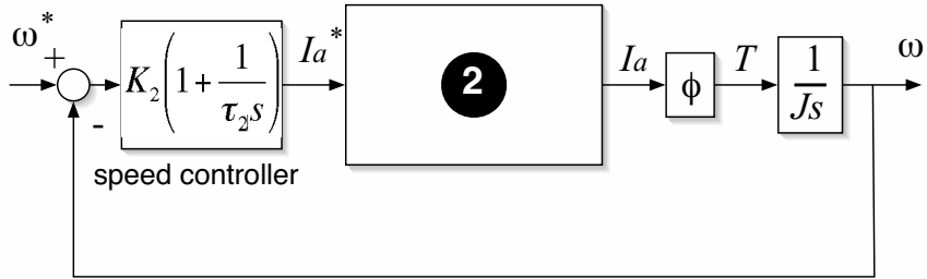
図 3: 速度制御部分の取り出し
