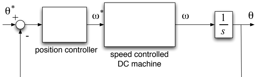
図 4: 位置制御系への展開
